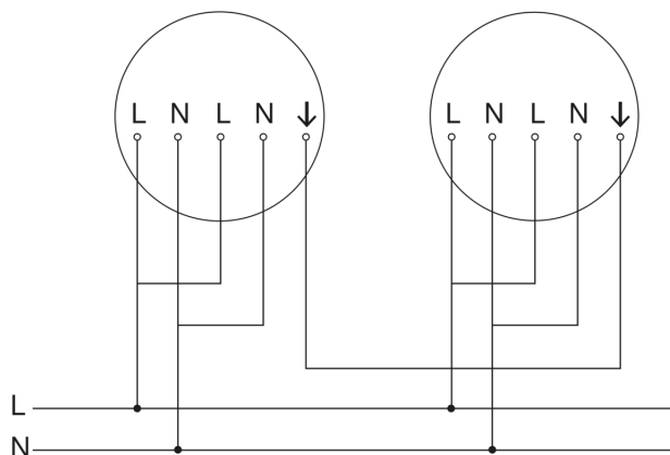
aansluitschema master/master
