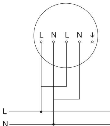
aansluitschema Master
